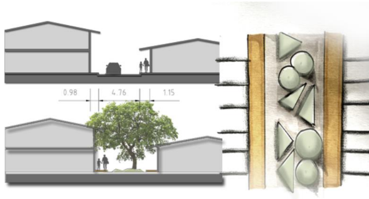
Gráfico 8 Perfil calle 2da_ realizado por estudiante.
